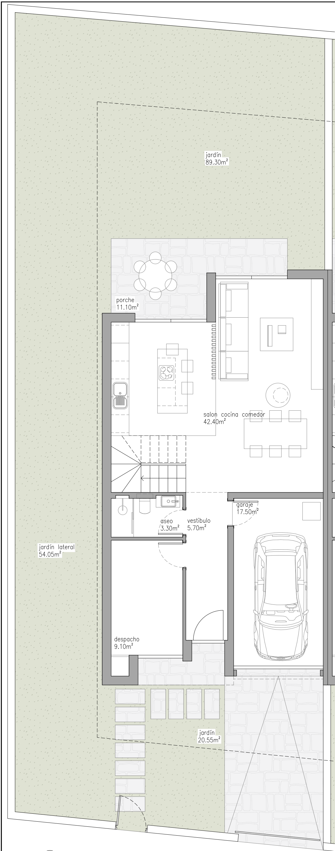
1 PLANTA BAJA Adosado 1
