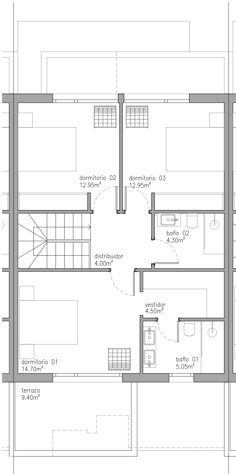
2 PLANTA PRIMERA Adosado 3
