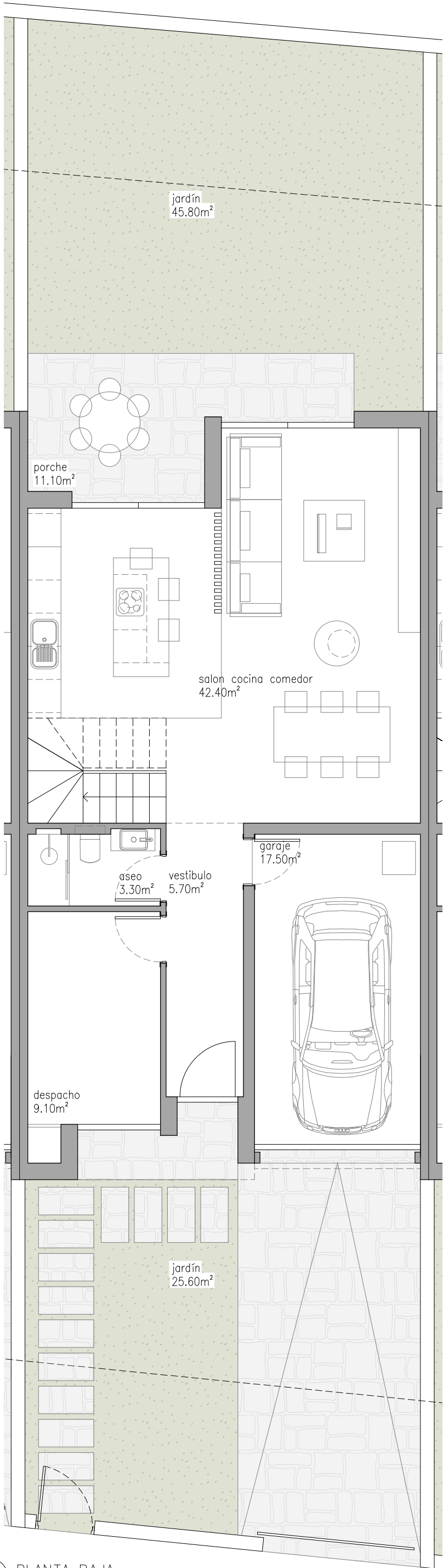
1 PLANTA BAJA Adosado 3
